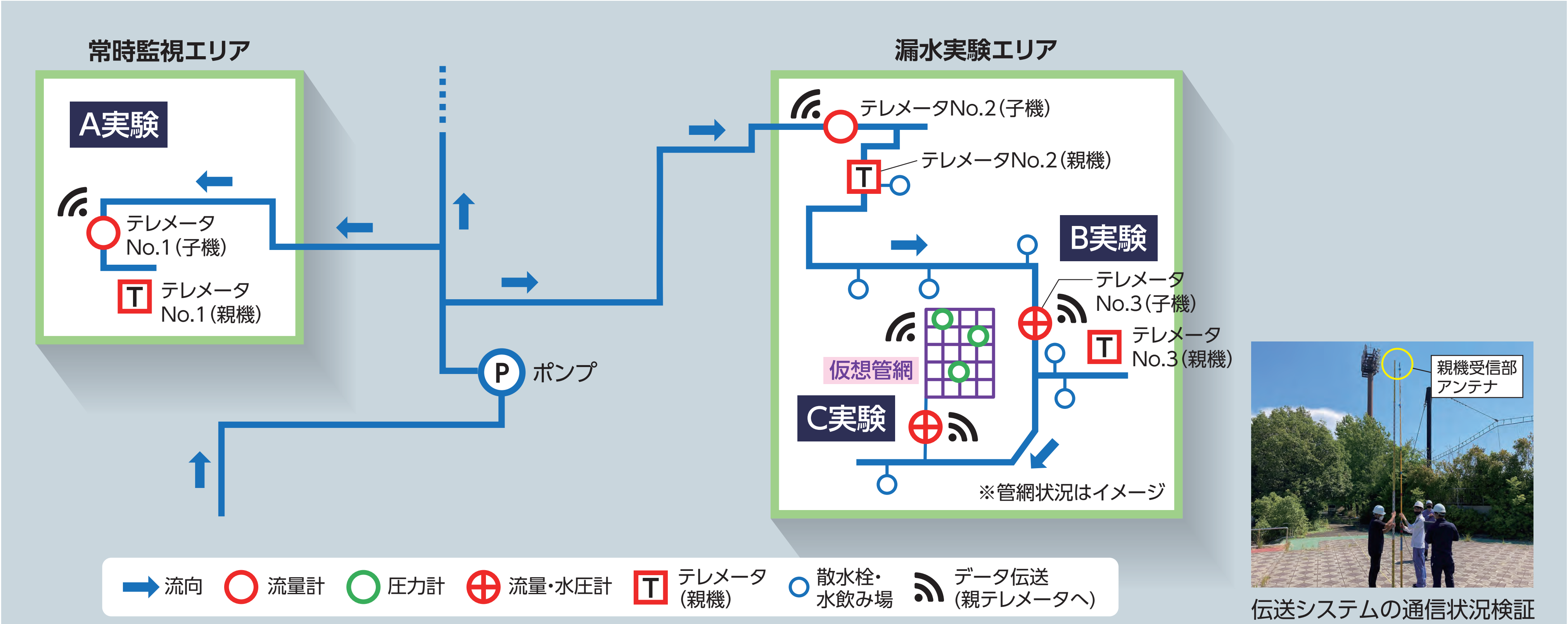
仮想管網
